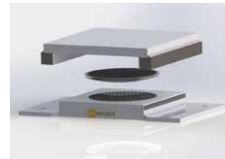
Apoyo esférico guiado MAURER, vista detallada
