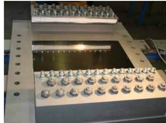
Apoyos esféricos antielevación MAURER
