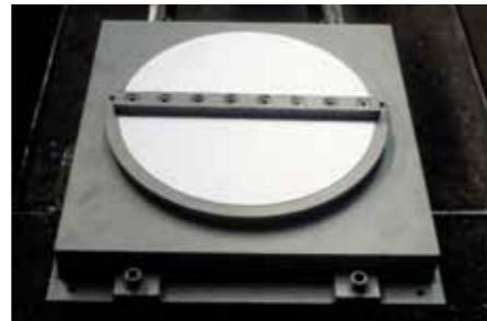
Apoyo tipo Pot MAURER
