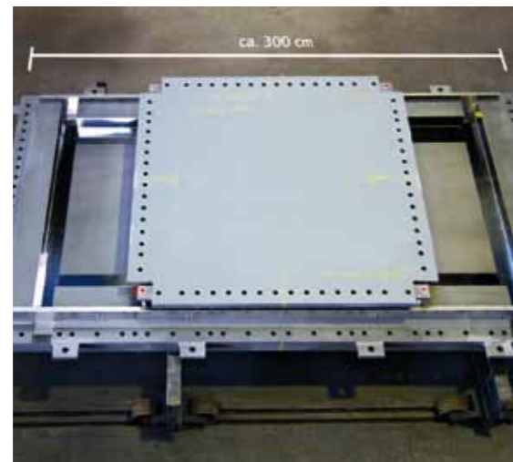
Llaves de cortante MAURER
